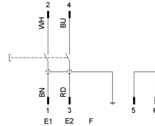
Schaltbild / Wiring diagram:
