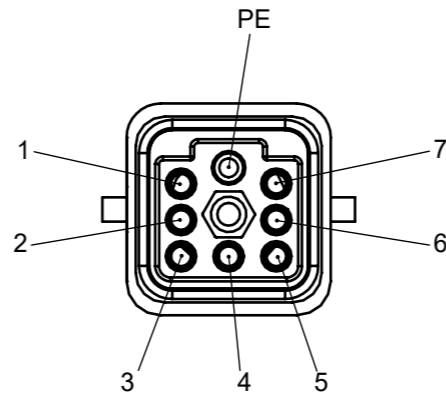
Polbild / Mating face Ansicht Steckseite / View of connection side 1:1
