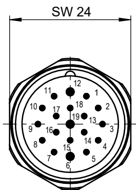
RC18 Ansicht Steckseite View plug connection
