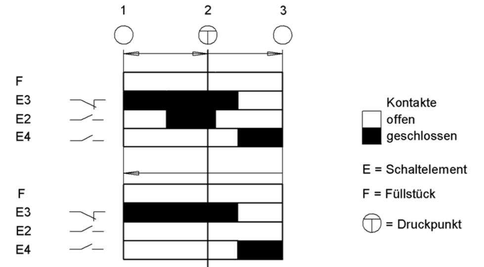
Schaltwegdiagramm
