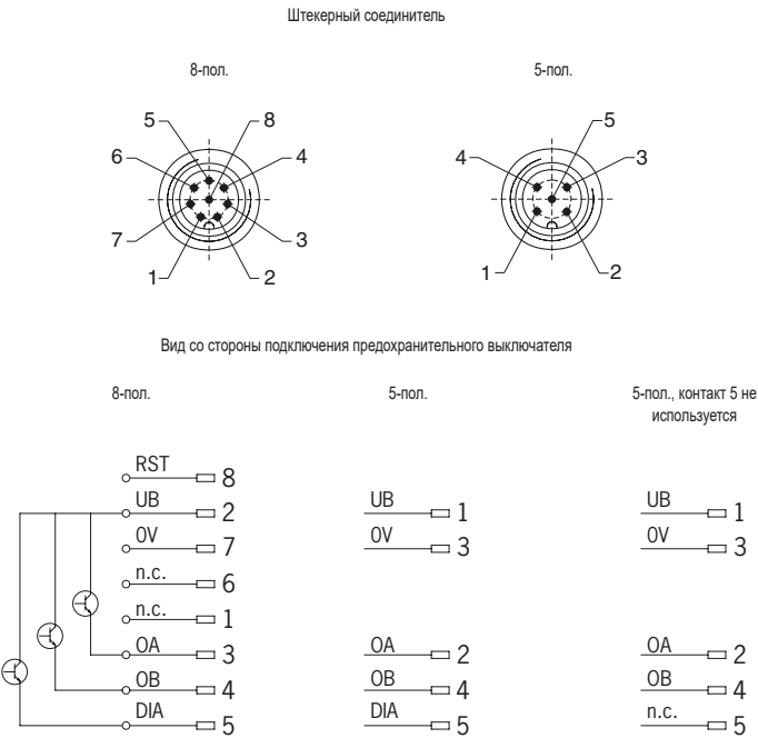
Рис. 1. Схема контактов штекерного соединителя предохранительного выключателя CES-AP-C01
