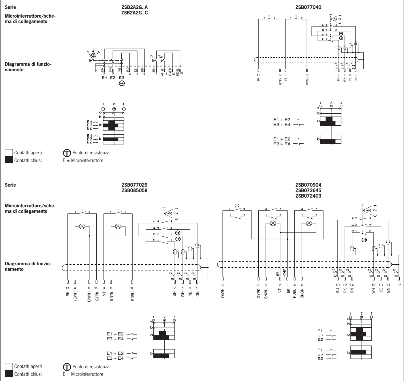
Fig. 2: Funzionamento degli elementi di comando e schemi di collegamento
