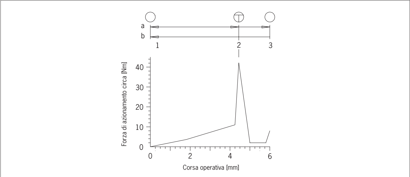
Fig. 3: Diagramma della forza di azionamento in funzione della corsa operativa
