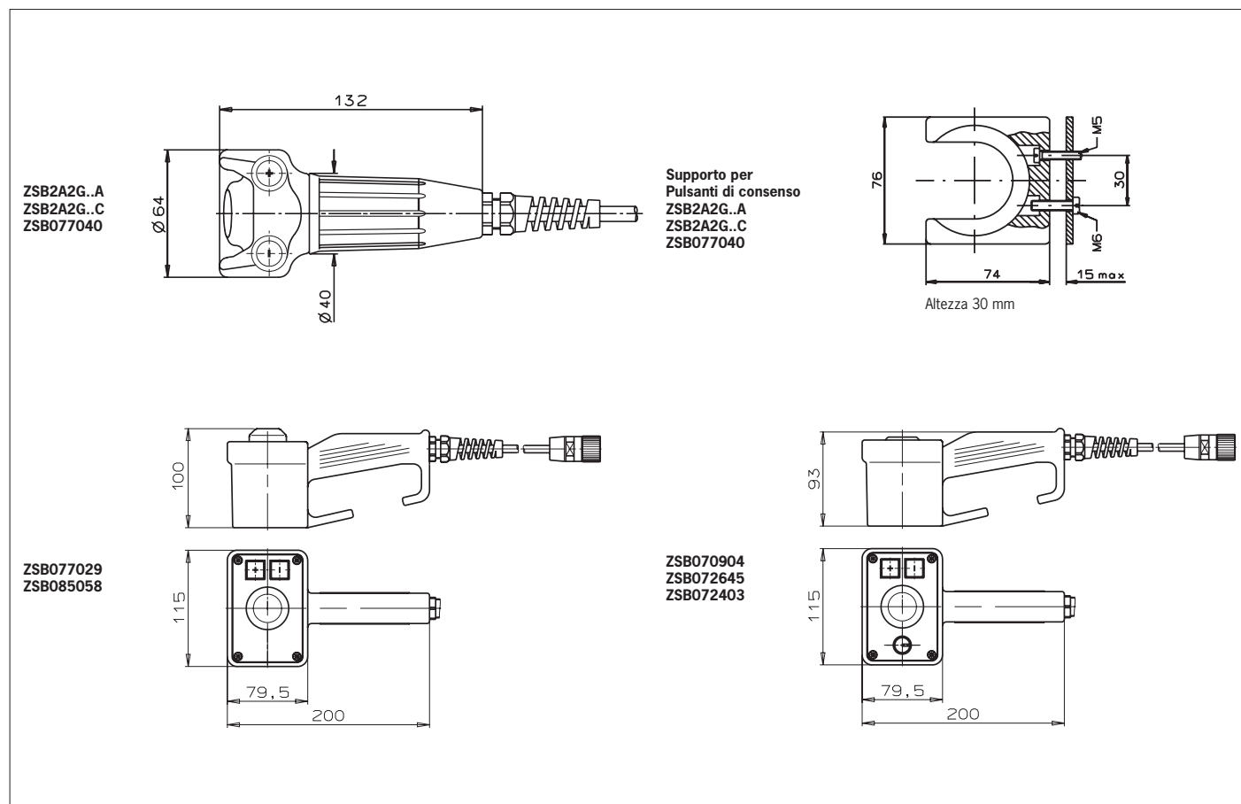
Fig. 1: Dimensioni del pulsante di consenso ZSA e del relativo supporto per pulsante di consenso ZSA
