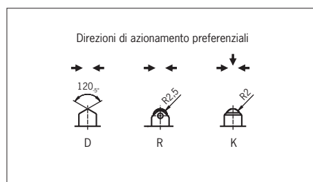
Fig. 2: Pulsanti e direzioni di azionamento
