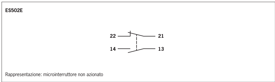
Fig. 1: Microinterruttori e schema di collegamento
