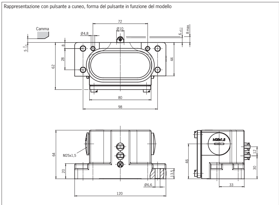
Fig. 2: Dimensioni GS...502-MC1806
