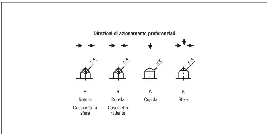
Fig. 3: Pulsanti e direzioni di azionamento
