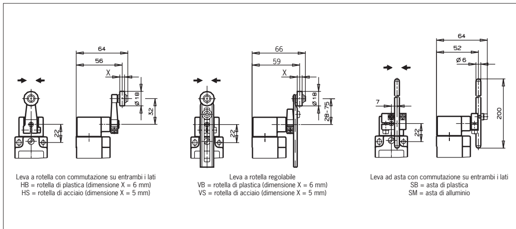
Fig. 7: Azionatore e direzioni di azionamento
