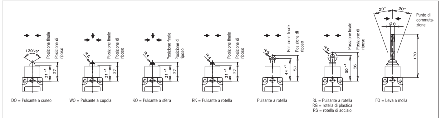
Fig. 6: Azionatore e direzioni di azionamento
