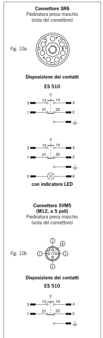
Fig. 10: Microinterruttori e collegamenti
