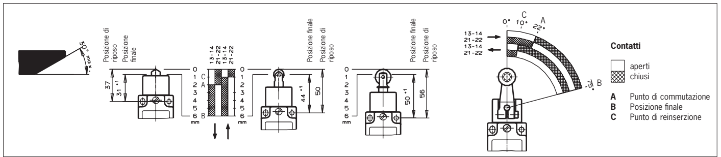
Fig. 5: Diagrammi di funzionamento
