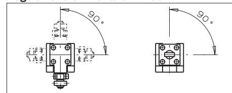
Fig. 3: Regolazione orizzontale
