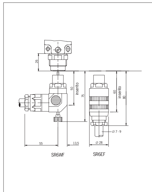
Fig. 9: Dimensioni NG2... con connettore SR6
