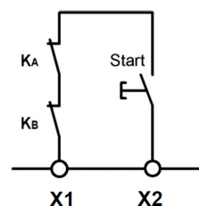
Fig. 6 : En cas d'utilisation de contacteurs ou de modules d'extension externes (p. ex. ESM-ES3..) à des fins de duplication ou de multiplication des contacts sur le ESM-2H2.., leurs contacts de signalisation à manœuvre positive (contacts d'ouverture) doivent être montés en série et reliés avec les connexions de la boucle de retour X1 et X2.
