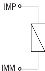
Fig. 6 : Exemple de raccordement avec connexion IMM
