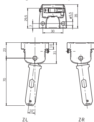
Languette articulée Z-L / Z-R
