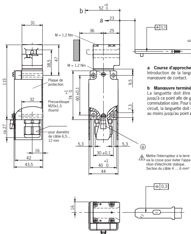
Fig. 3 : Dimensions NZ1VZ...EX
