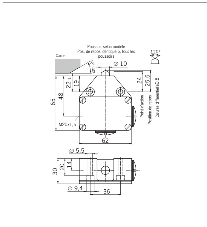
Fig. 4 : Dimensions N10
