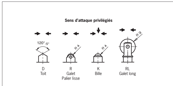
Fig. 3 : Poussoirs et sens d'attaque
