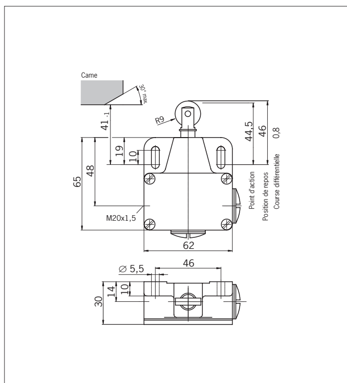
Fig. 7 : Dimensions N11 avec poussoir à galet long
