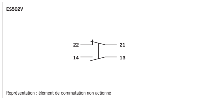
Fig. 2 : Élément de commutation et affectation des broches
