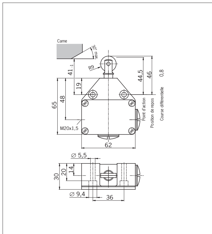
Fig. 5 : Dimensions N10 avec poussoir à galet long
