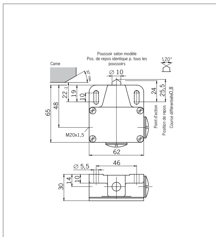
Fig. 6 : Dimensions N11
