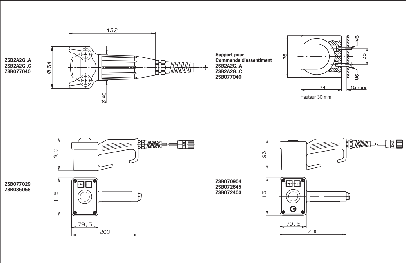
Fig. 1 : Dimensions commande d'assentiment ZSA et support pour commande d'assentiment ZSA
