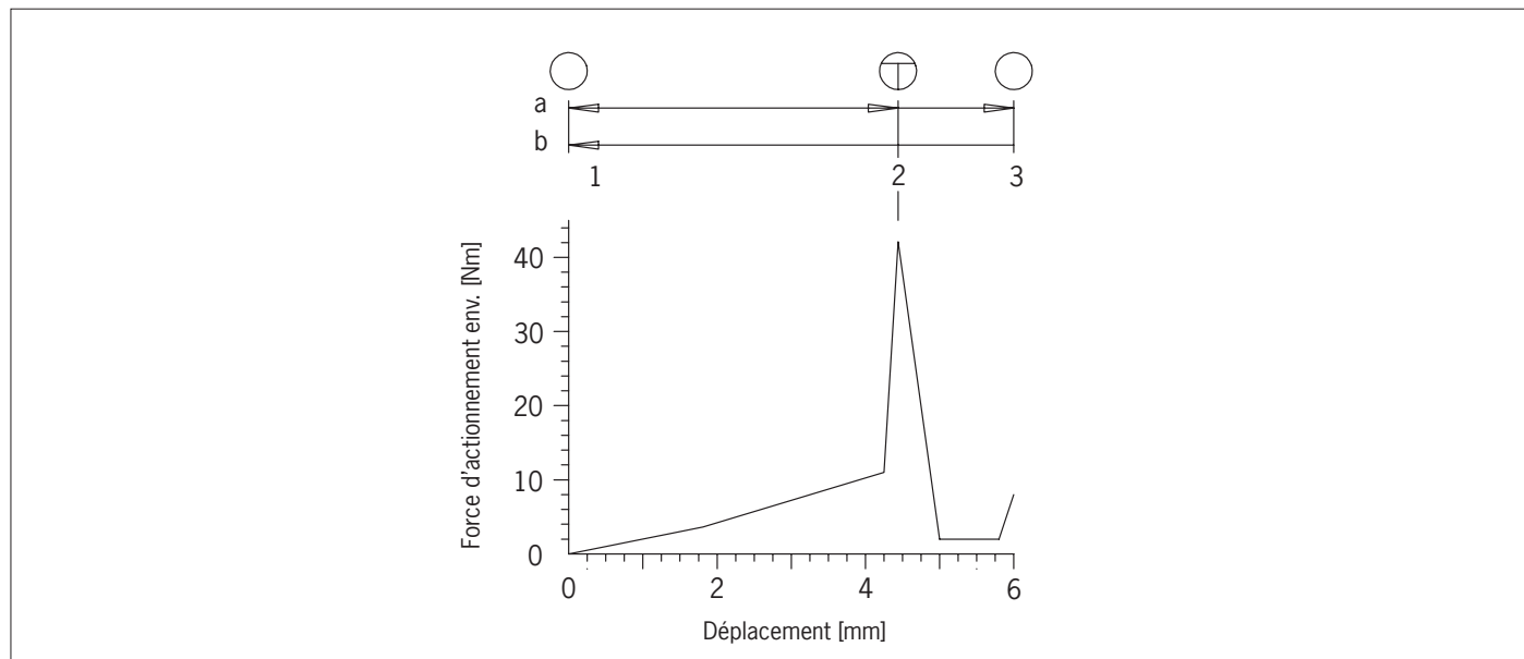
Fig. 3 : Diagramme force d'actionnement en fonction du déplacement
