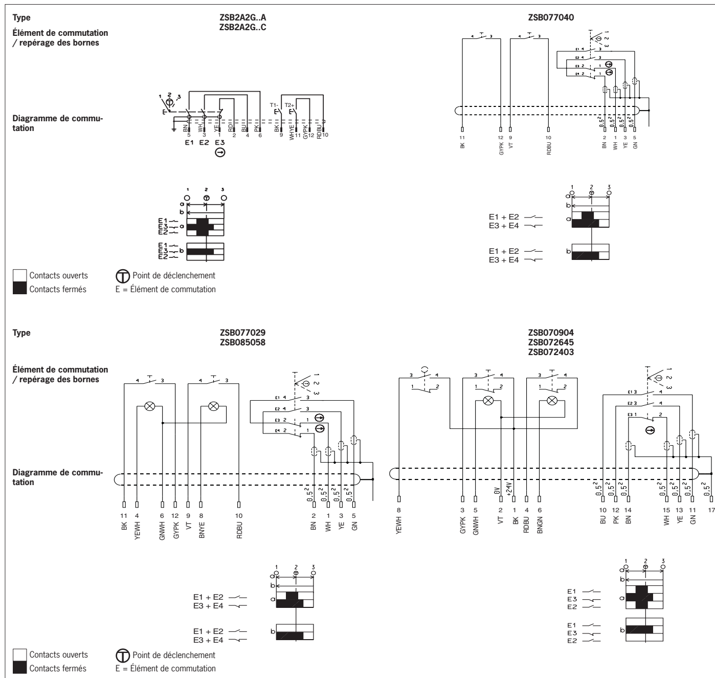
Fig. 2 : Fonction des éléments de commutation et repérage des bornes
