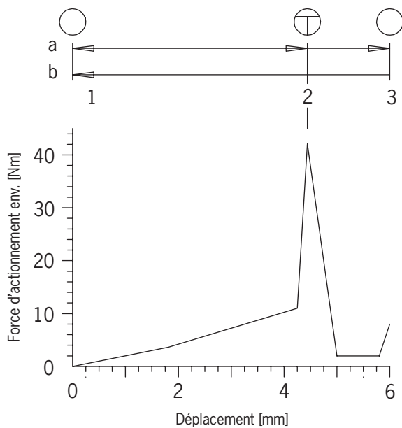
Fig. 4 : Diagramme force d'actionnement en fonction du déplacement
