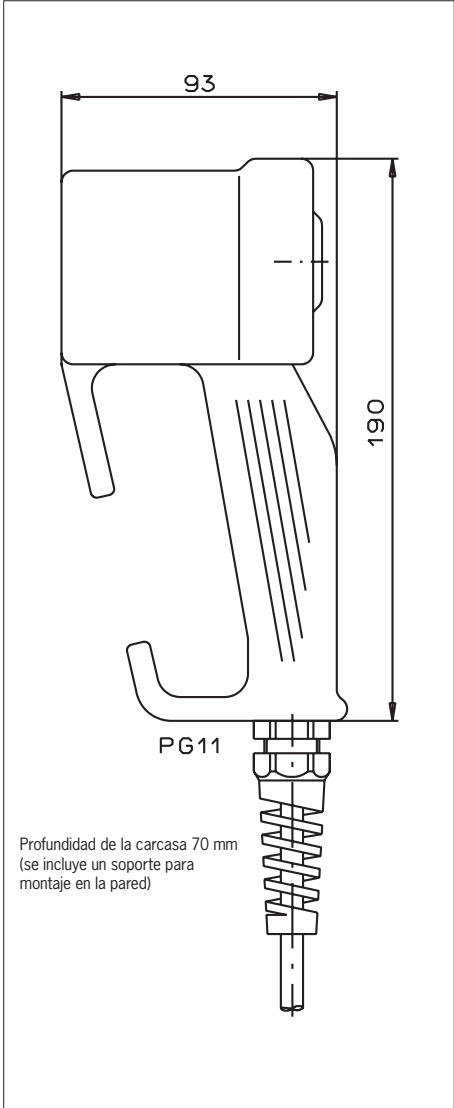
Fig. 3: Plano de dimensiones del pulsador de validación ZSR
