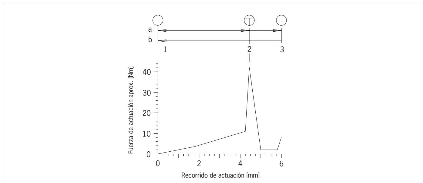
Fig. 3: Diagrama de la fuerza de actuación en función del recorrido de actuación
