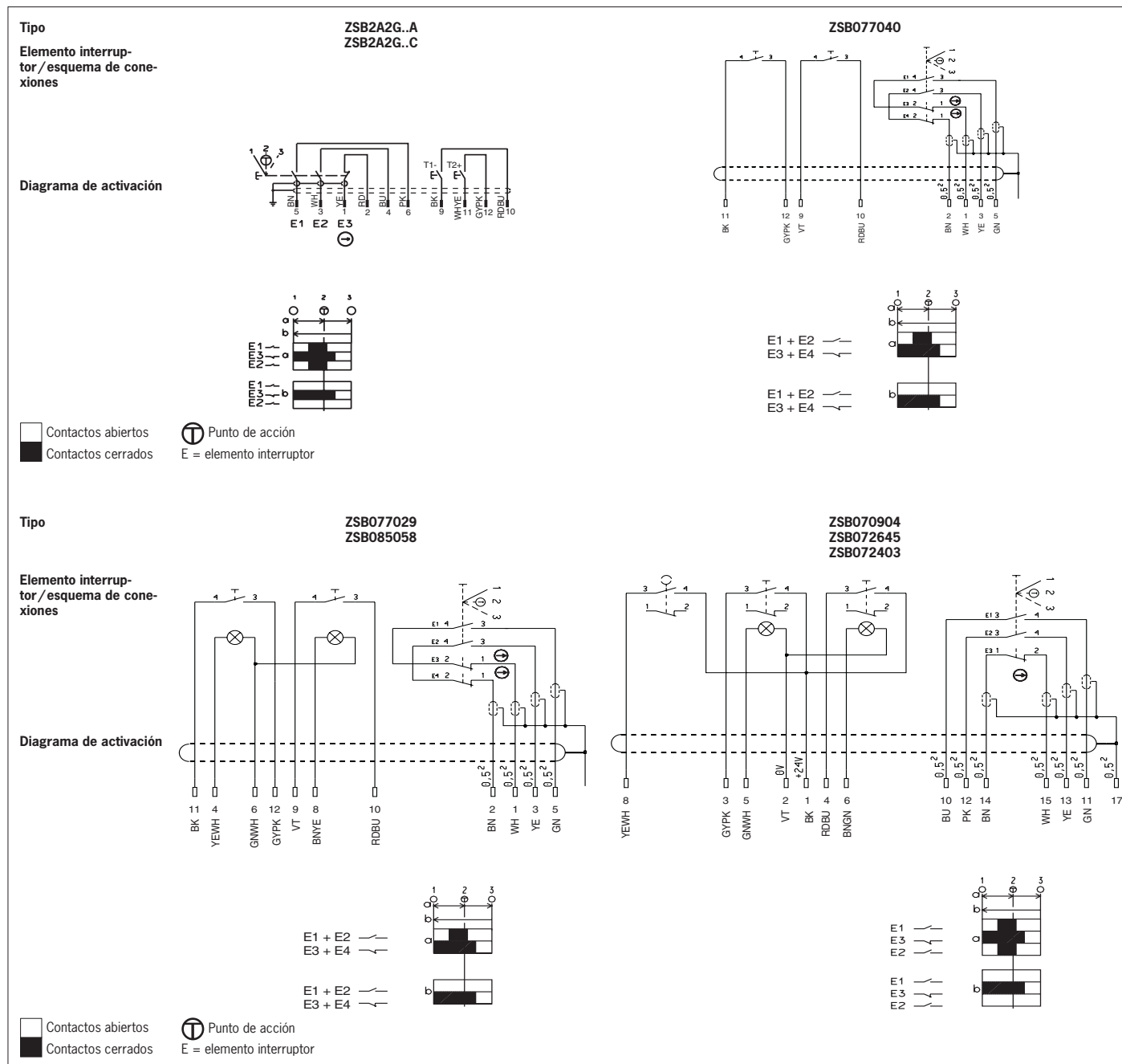
Fig. 2: Funcionamiento de los elementos interruptores y esquemas de conexiones
