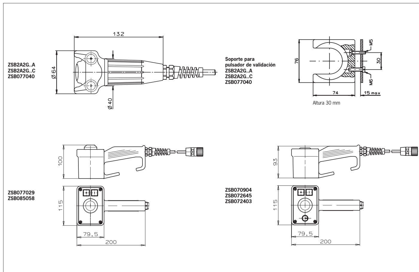
Fig. 1: Plano de dimensiones del pulsador de validación ZSA y su respectivo soporte
