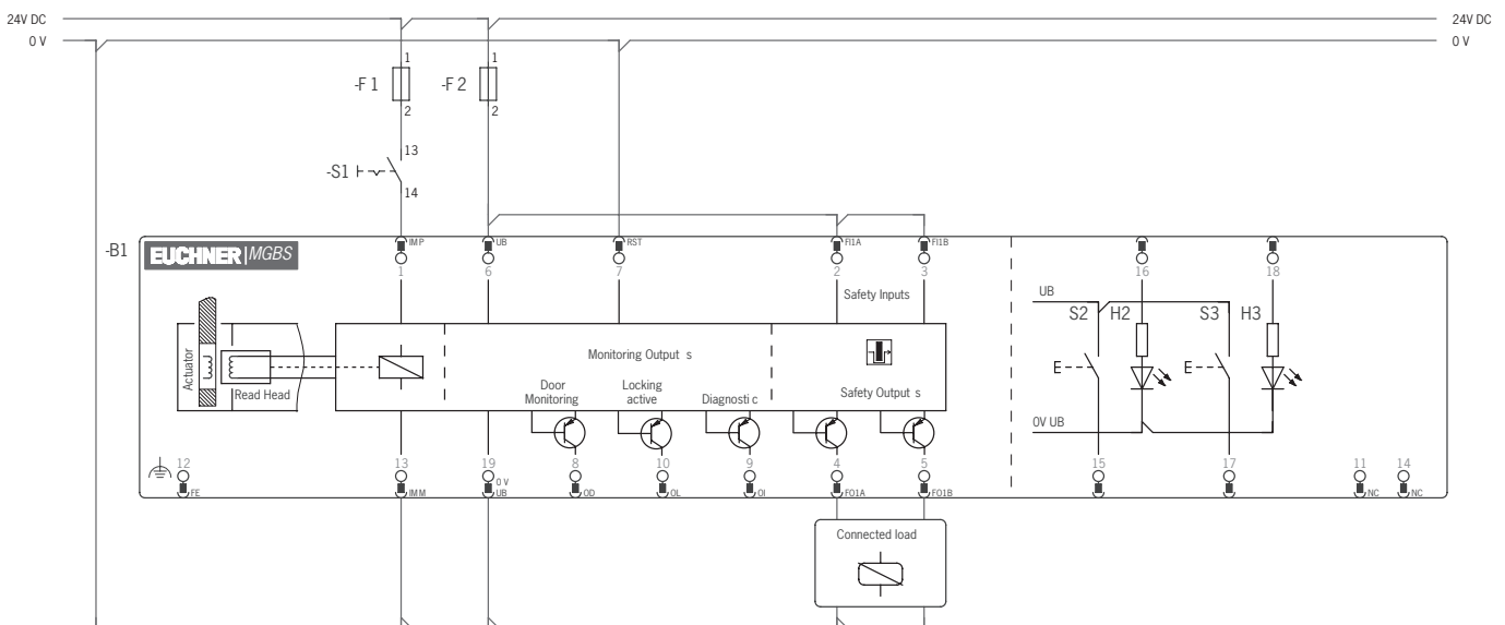
Fig. 5: Ejemplo de conexión para funcionamiento independiente, versión con conector M23
