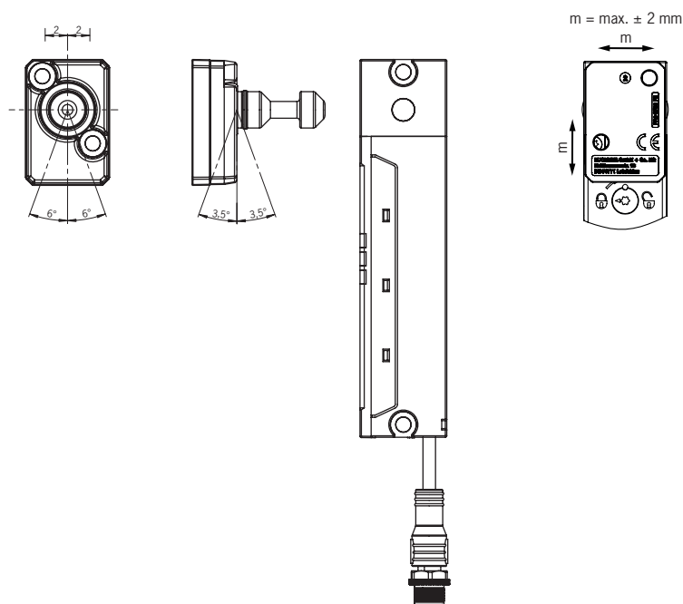
Fig.5: Movimiento máximo del actuador y holgura central máxima
