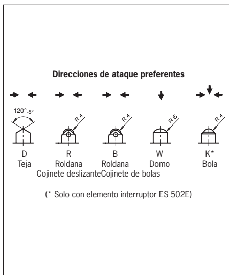
Fig. 4: Accionadores y direcciones de ataque
