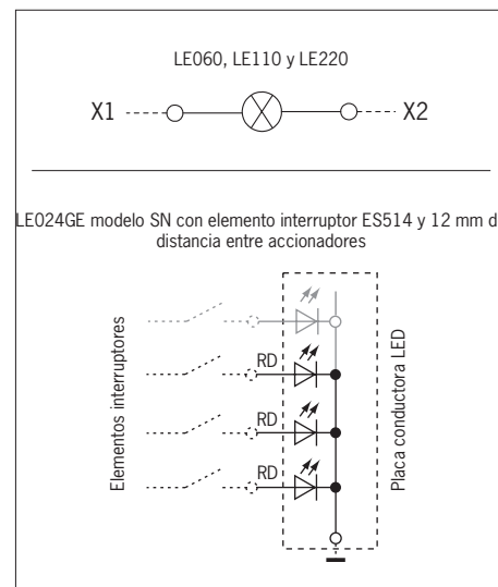
Fig. 5: Conexión de indicadores LED
