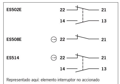
Fig. 1: Elementos interruptores y asignación de contactos
