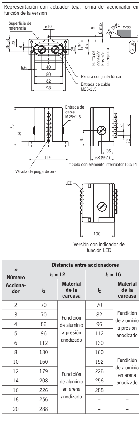
Fig. 3: Plano de dimensiones GS...
