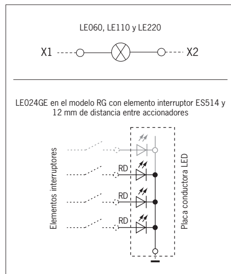
Fig. 7: Conexión de indicadores LED
