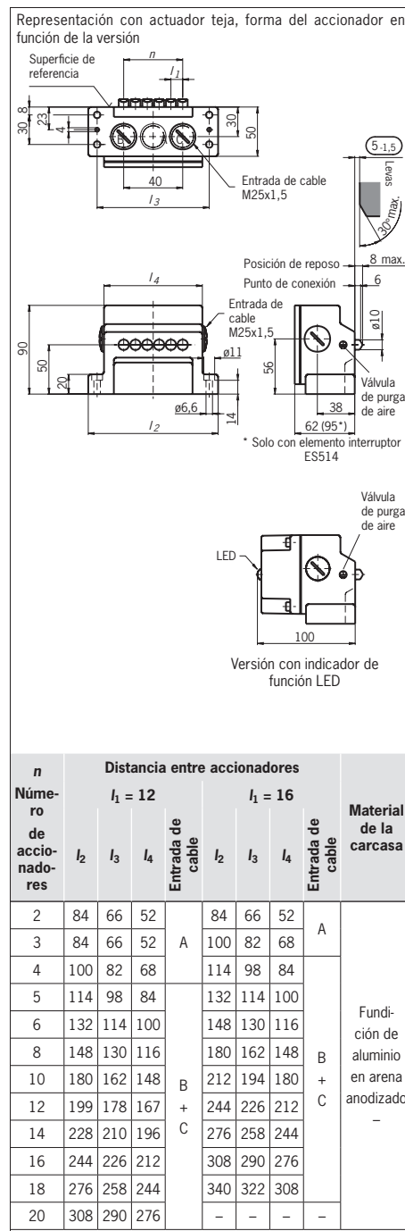
Fig. 4: Plano de dimensiones GL...
