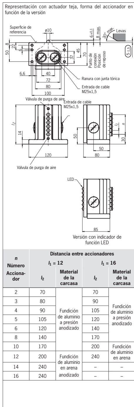
Fig. 2: Plano de dimensiones RG...
