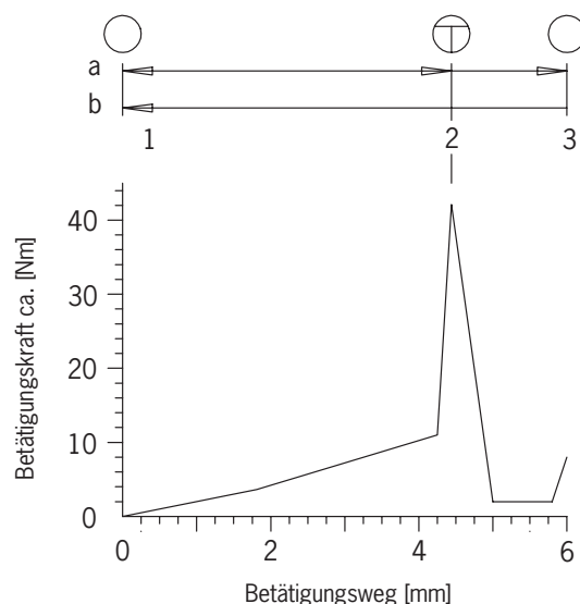
Bild 3: Diagramm Betätigungskraft in Abhängigkeit vom Betätigungsweg
