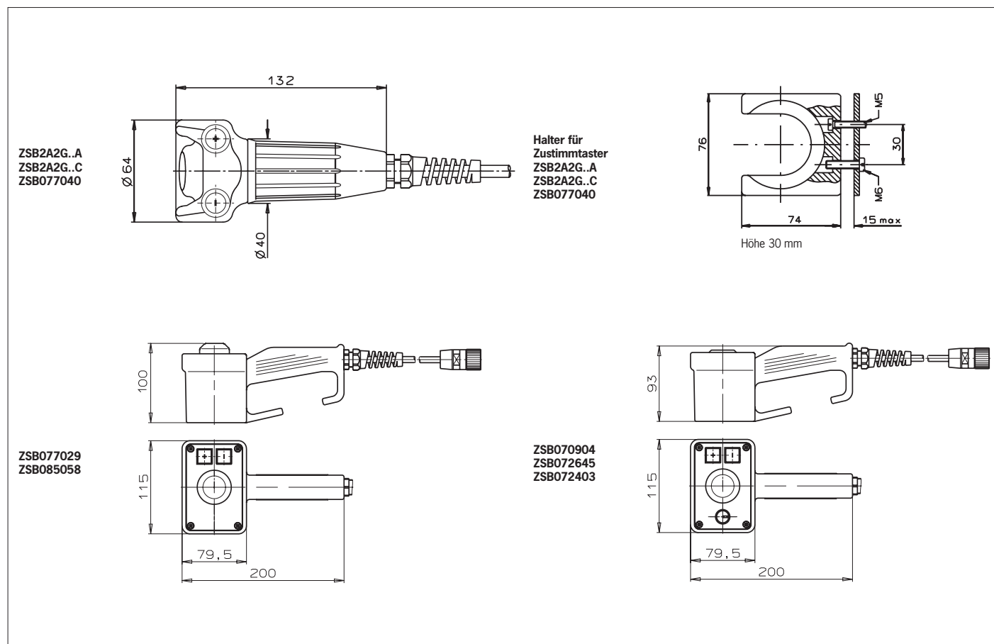
Bild 1: Maßzeichnung Zustimmtaster ZSA und Halter für Zustimmtaster ZSA
