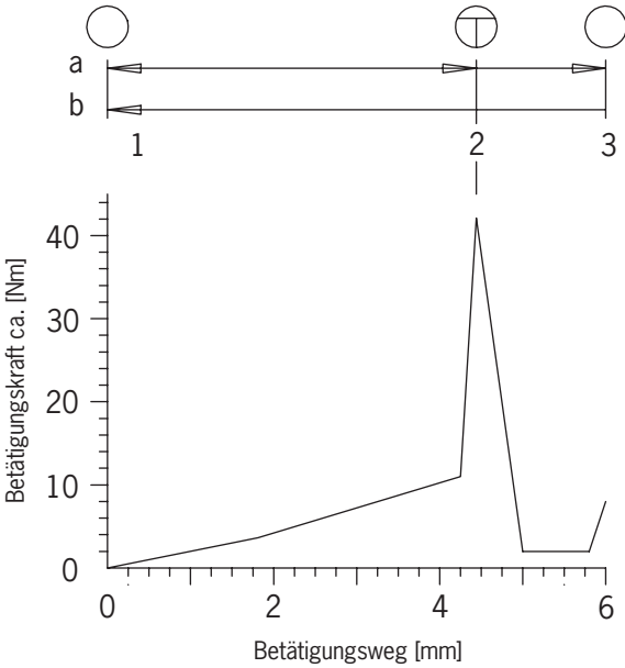
Bild 4: Diagramm Betätigungskraft in Abhängigkeit vom Betätigungsweg
