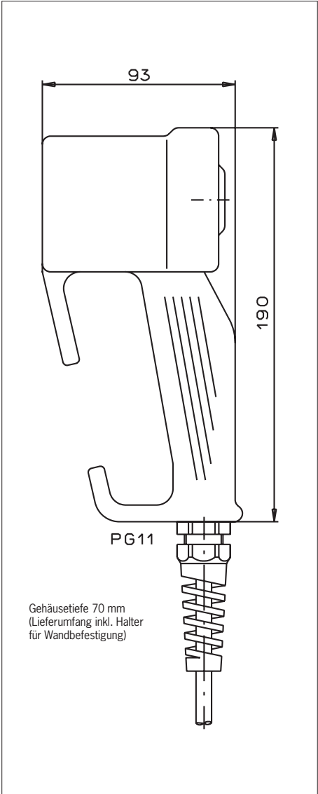
Bild 3: Maßzeichnung Zustimmtaster ZSR
