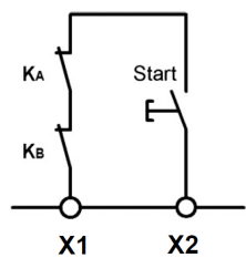
Bild 5: Verdrahtung des ESM-2H2.. mit Zweihandtaster (Öffner-/Schließkontakt)
