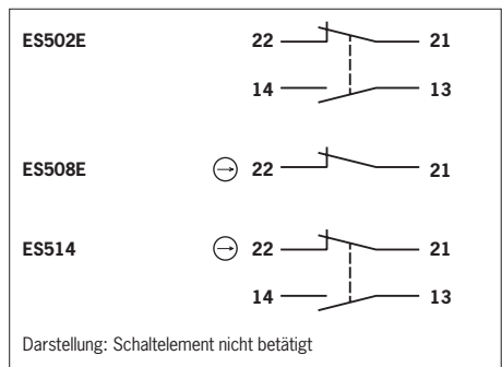
Bild 1: Schaltelemente und Anschlussbelegung
