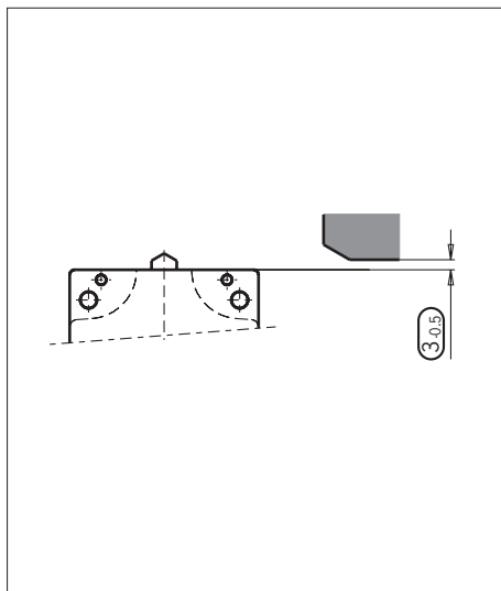
Bild 3: Montage SN...-508 und SN...-514 für Sicherheitschaltkreise
