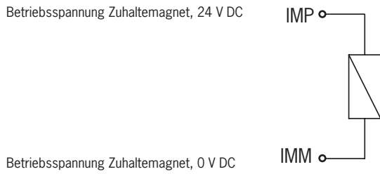
Bild 8: Anschlussbeispiel mit Anschluss IMM
